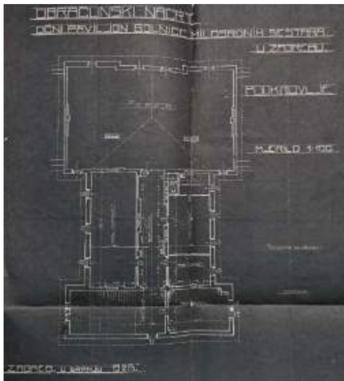
1903.g. tlocrt potkrovlja (Klinika za očne bolesti)
