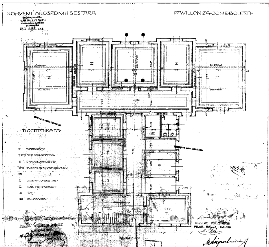
1903.g. tlocrt 2.kata osnovne zgrade (Klinika za očne bolesti)
