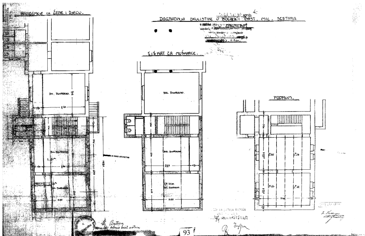
1913.g. dogradnja osnovne zgrade (Klinika za kožne i spolne bolesti)-tlocrti
