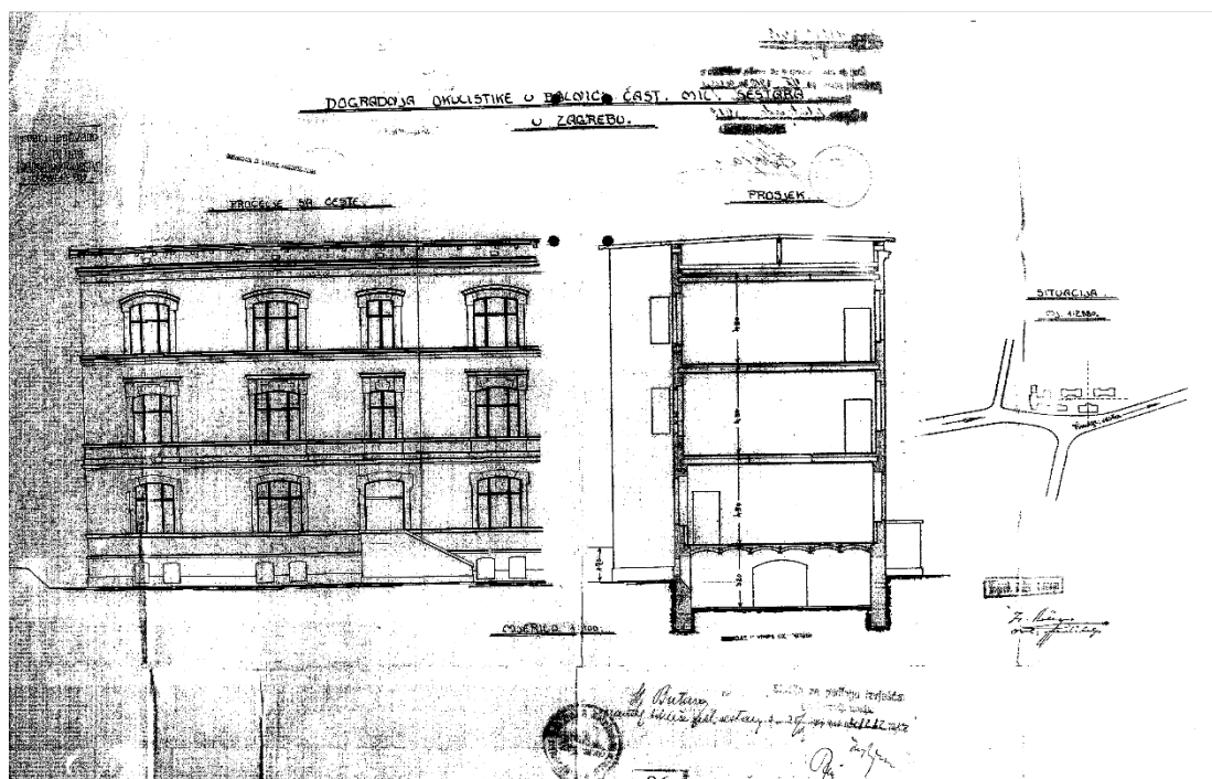
1913.g. dogradnja osnovne zgrade (Klinika za kožne i spolne bolesti)-pročelje i presjek
