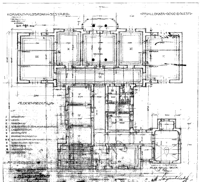
1903.g. tlocrt prizemlja osnovne zgrade (Klinika za očne bolesti)
