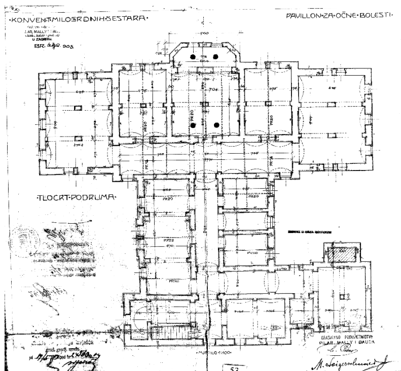
1903. Tlocrt podruma osnovne zgrade (Klinika za očne bolesti)
